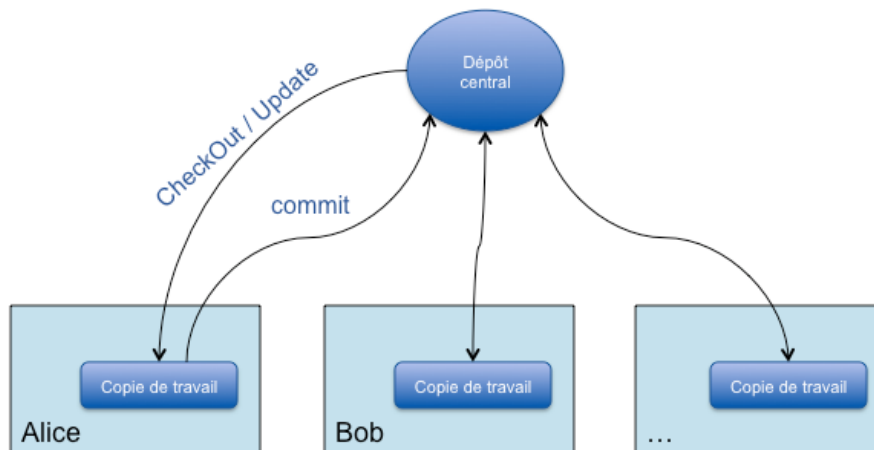
Figure 1: Fonctionnement classique d'un gestionnaire de version (centralisé) 2
